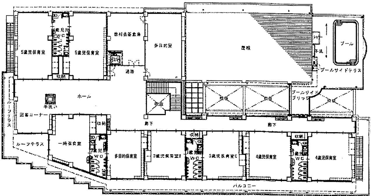
2階平面図
